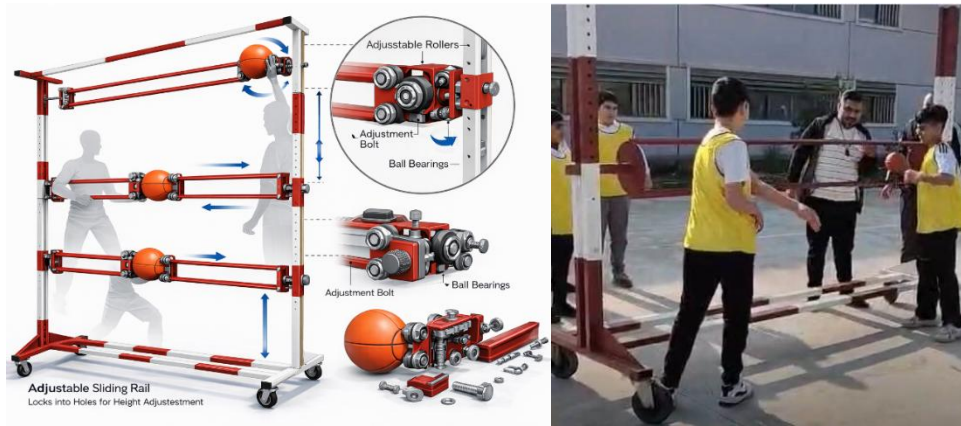
شكل (12) طريقة التمرين على الجهاز
